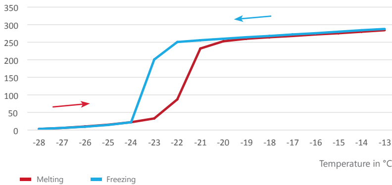
Enthalpy (J/g)
