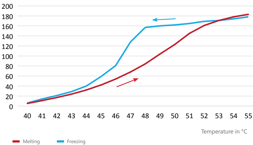
Enthalpy (J/g)
