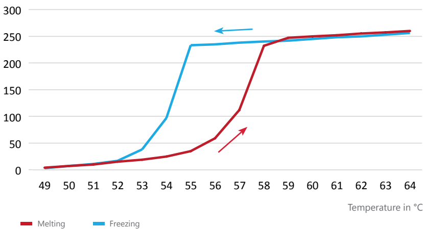
Enthalpy (J/g)
